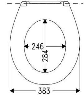
Gesamtlänge: 431 mm
