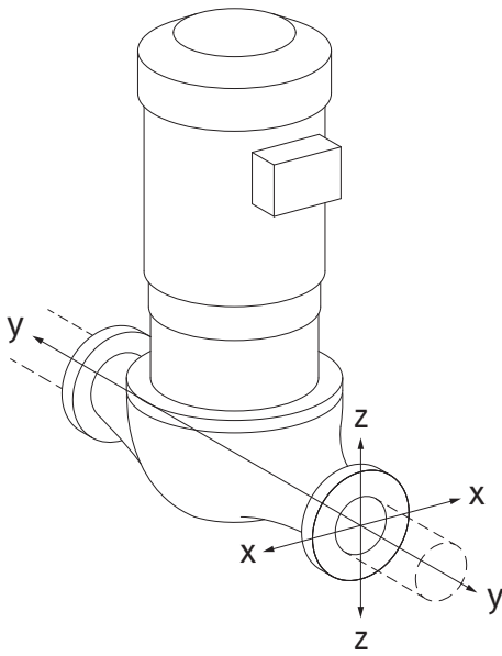
Fig. 20: Belastingsgeval 16A, EN ISO 5199, bijlage B
