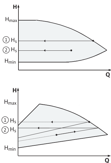
Fig. 32: Regeling \Delta p-c/\Delta p-v
