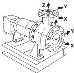
Fig. 22: Belastingsgeval 1A
