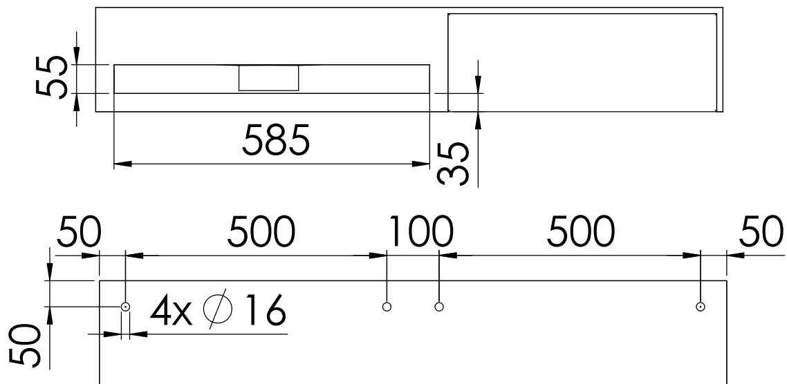
Schnitt B-B
