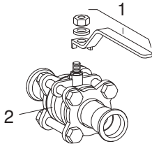
Bilde 1: Oppbygging Geberit Mapress kuleventil
