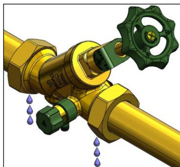
Funktionsprüfung n.i.O.
