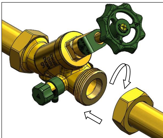
Montageschritt 4
