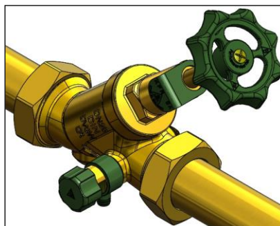
Funktionsprüfung i.O.
