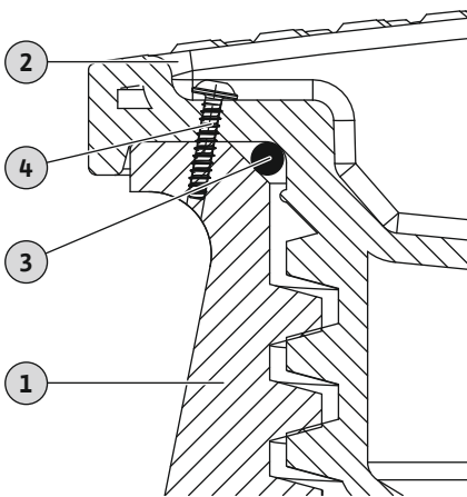
Fig. 19: Installare e fissare la copertura del pozzetto
