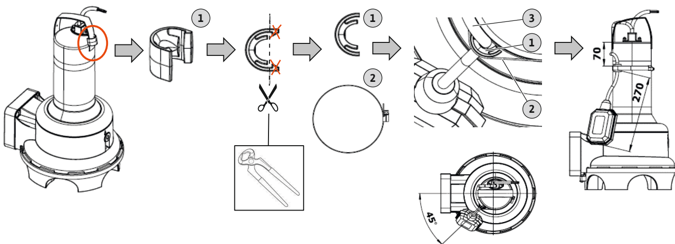
Fig. 15: Rexa UNI: Float switch cable length
