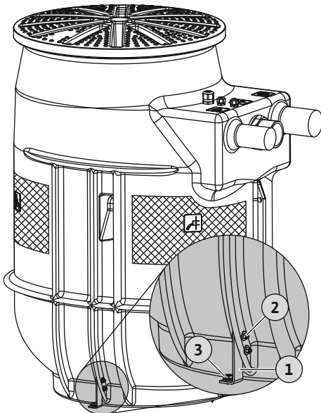
Fig. 4: Pumpenschacht aufstellen
