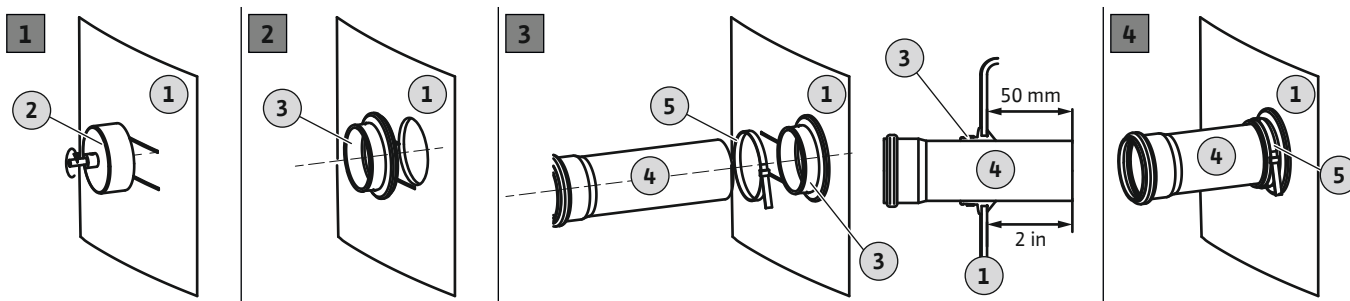
Fig. 8: Zulauf anschließen
