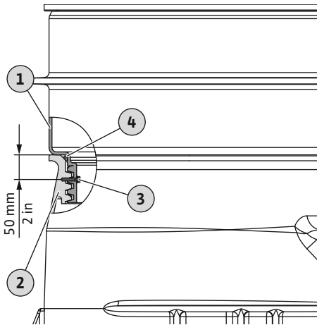
Fig. 12: Schachtverlängerung montieren
