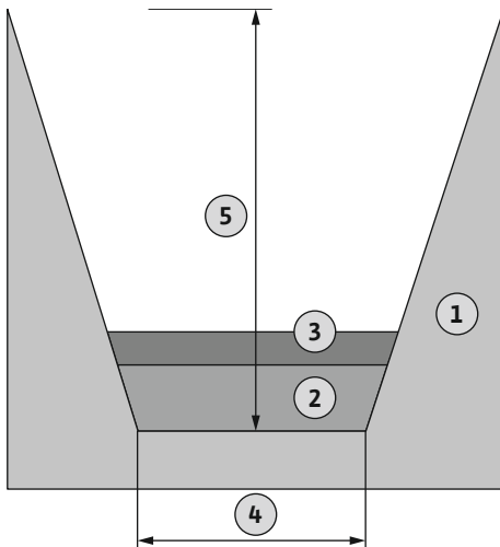
Fig. 5: Grube ausheben
