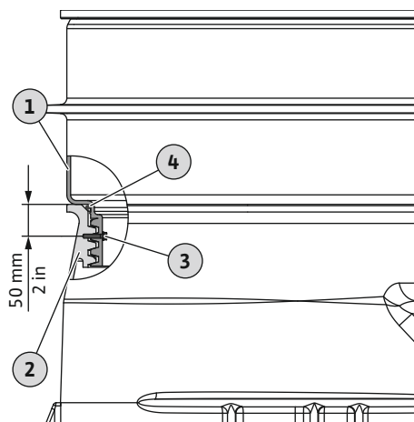
Fig. 12: Montare la prolunga del pozzo
