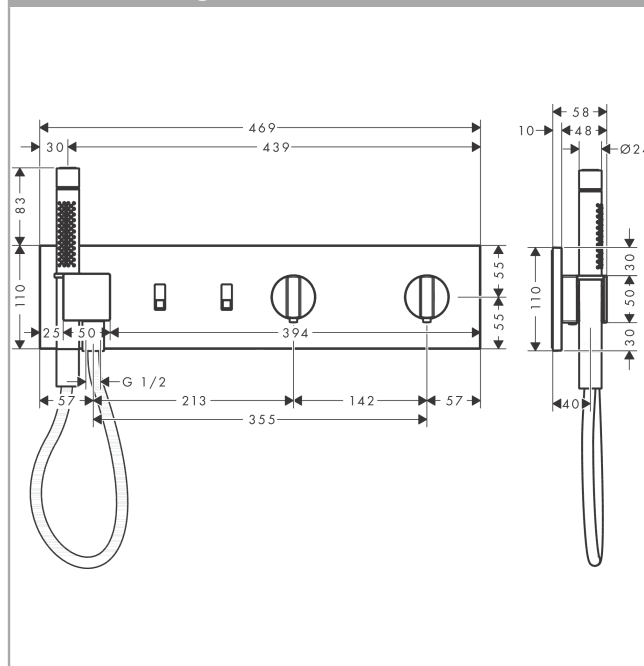
Maßzeichnung
