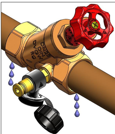
Funktionsprüfung n.i.O.
