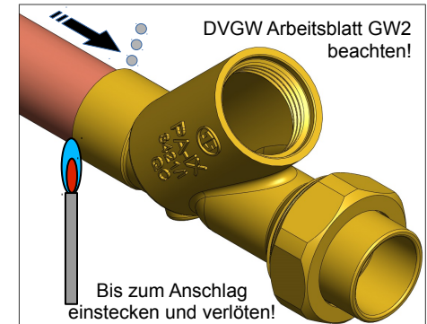
Montageschritt 4
