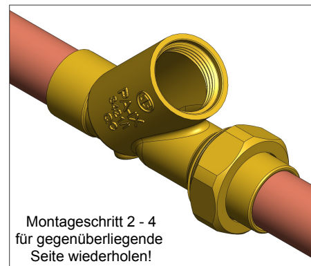
Montageschritt 5
