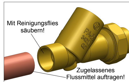
Montageschritt 3
