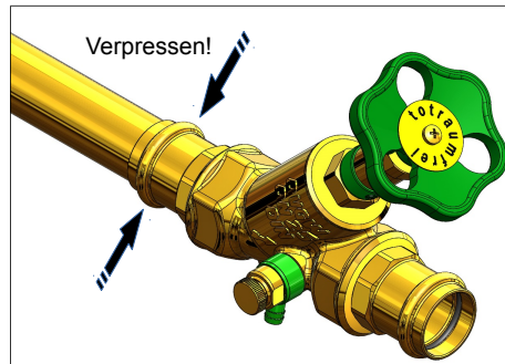
Montageschritt 4
