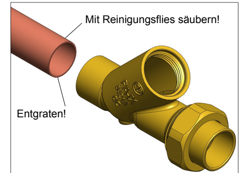
Montageschritt 4
