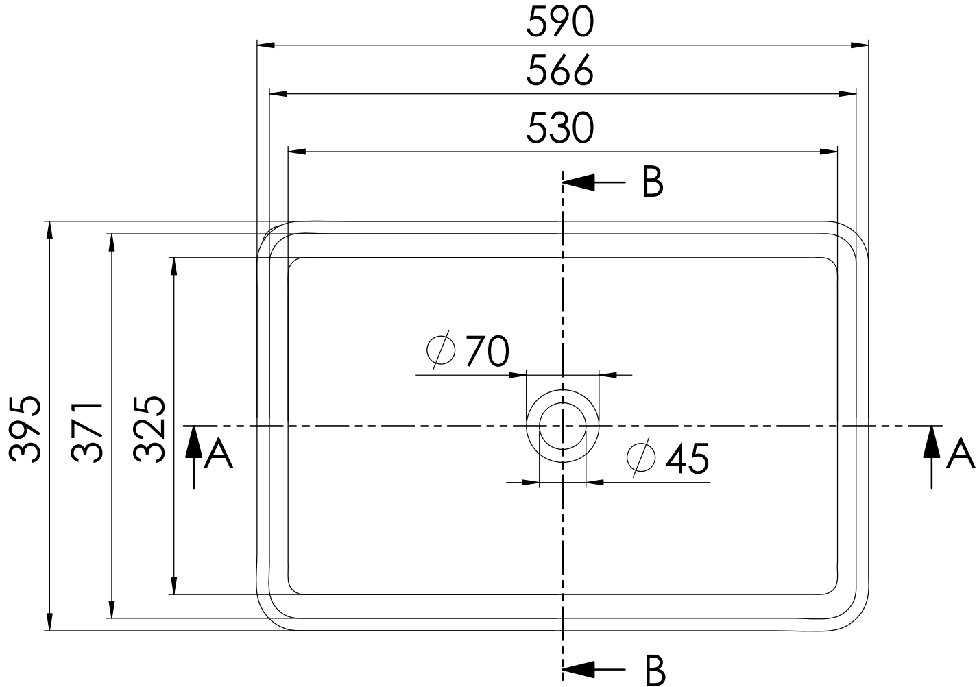
SCHNITT A-A
