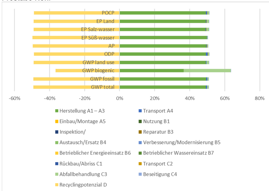
Abbildung 3: Prozentuale Anteile der Module an ausgewählten Umweltwirkungsindikatoren
