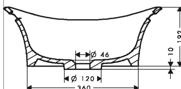
取付穴開口寸法
