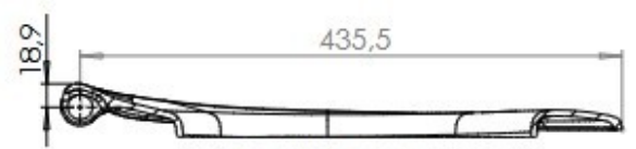
SCHNITT C-C
