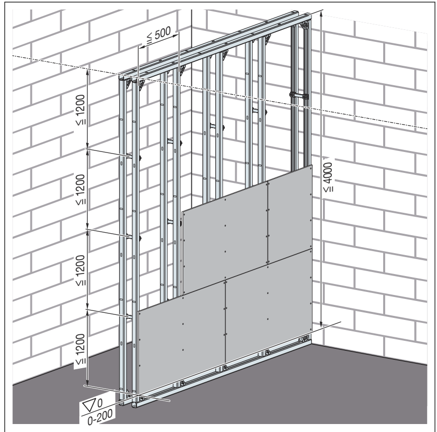
Steptec-Ständerwerke einlagig beplanken.
