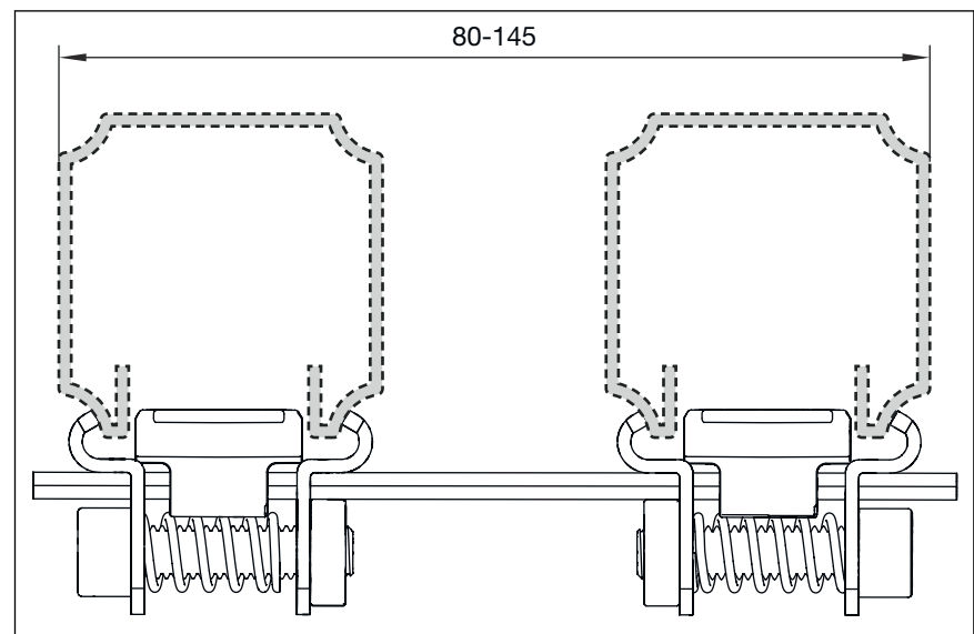
Abb. 2: Maßzeichnung
