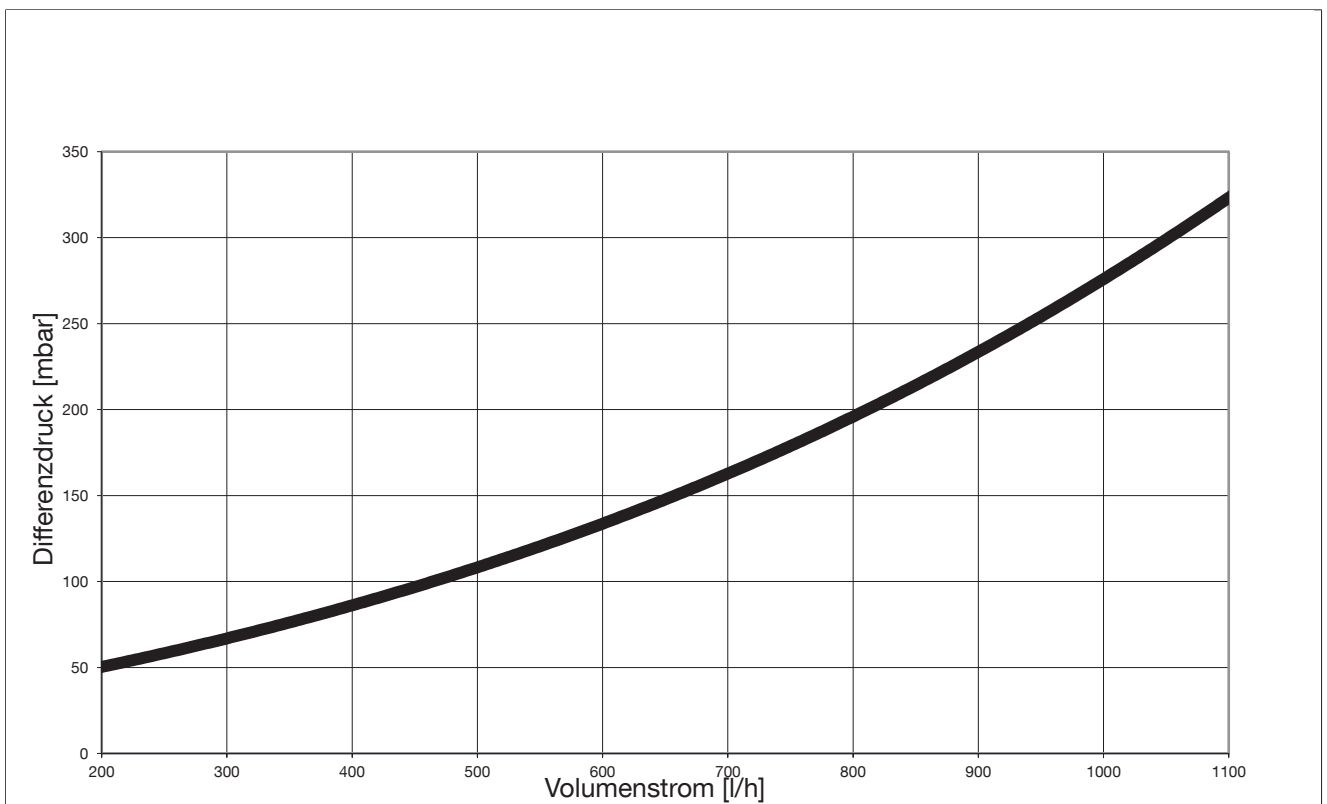
Abb. 5: Druckverlust Sekundärkreis Regudis H
