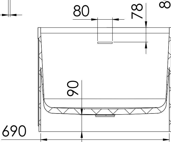
Schnitt B-B
