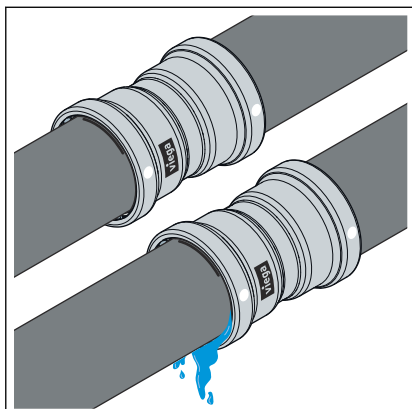
Abb. 9: SC-Contur
