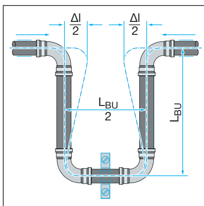
Abb. 6: Biegeschenkel U-Form
