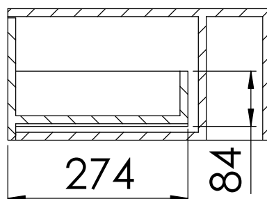
SCHNITT B-B
