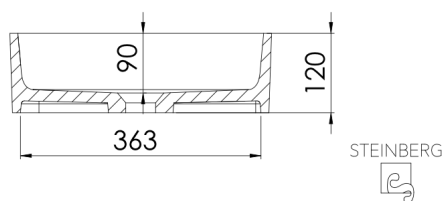
SCHNITT B-B
