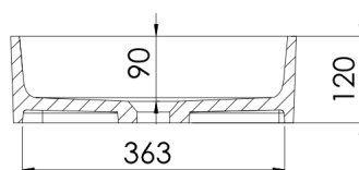
SCHNITT B-B
