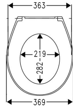
Gesamtlänge: 442 mm
