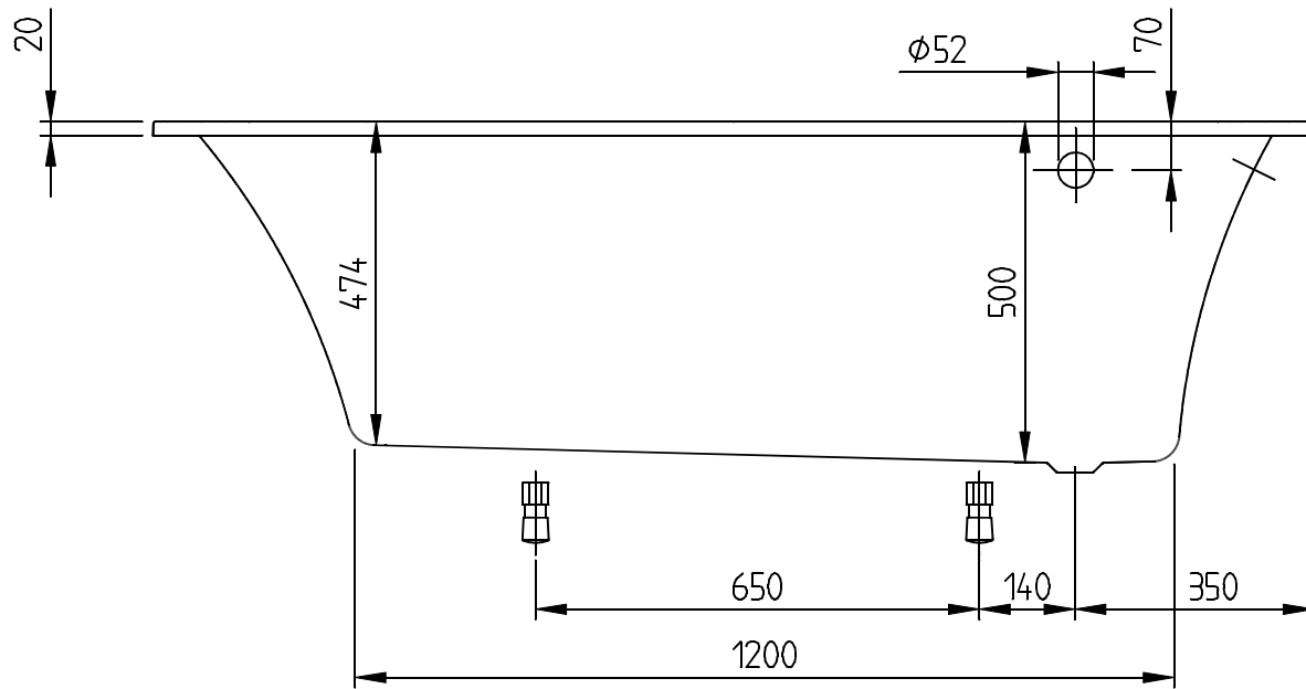
A-A
