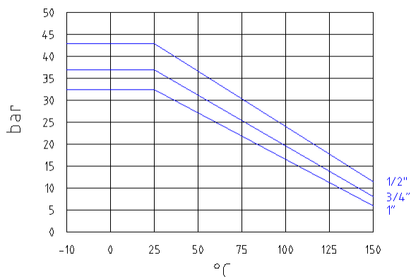
Druck-Temperatur-Diagramm
