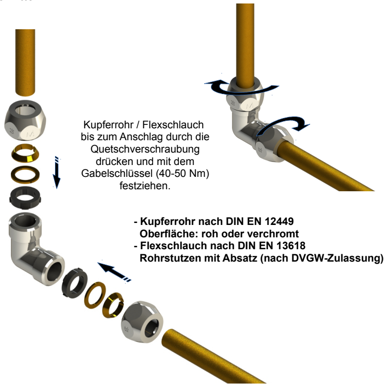
Montagebeispiel für Art. 8393
