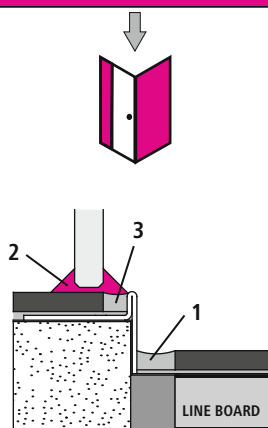
2 Versiegelung / Scellement / Sealing / Siliconen-kitnaad / Sigillatura / Sellado / Uszczelnienie zewnętrzne / Uzavírací náter / Tesniaca hmota / Герметик / 封闭膜 / Försigling / Försigling / Elzárás
