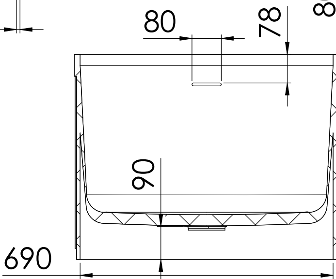
Schnitt B-B
