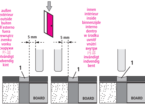
2 Versiegelung / Scellement / Sealing / Siliconen-kitnaad / Sigillatura / Sellado / Uszczelnienie zewnętrzne / Uzavirací nátěr / Tesniaca hmota / Герметик / 封闭膜 / Försegling / Försegling / Elzárás
