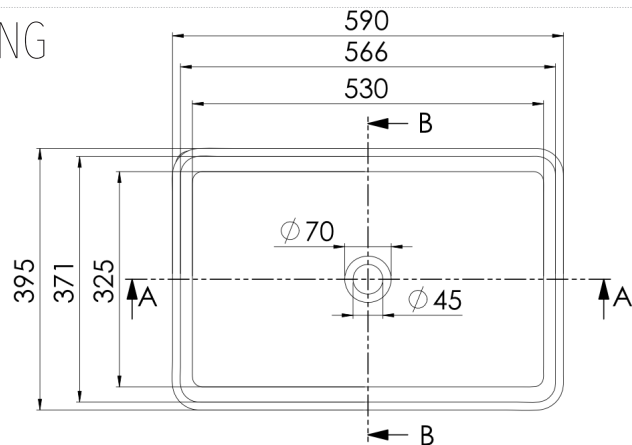
SCHNITT A-A
