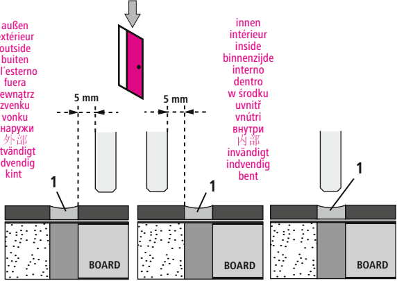
2 Versiegelung / Scellement / Sealing / Siliconen-kitnaad / Sigillatura / Sellado / Uszczelnienie zewnętrzne / Uzavirací nátěr / Tesniaca hmota / Герметик / 封闭胶 / Försegling / Forsegling / Elzárás
