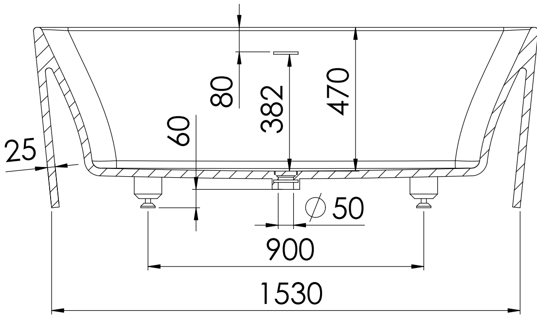
SCHNITT B-B
